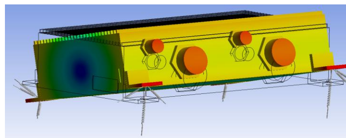
Одна из форм колебаний виброзащищаемого блока
