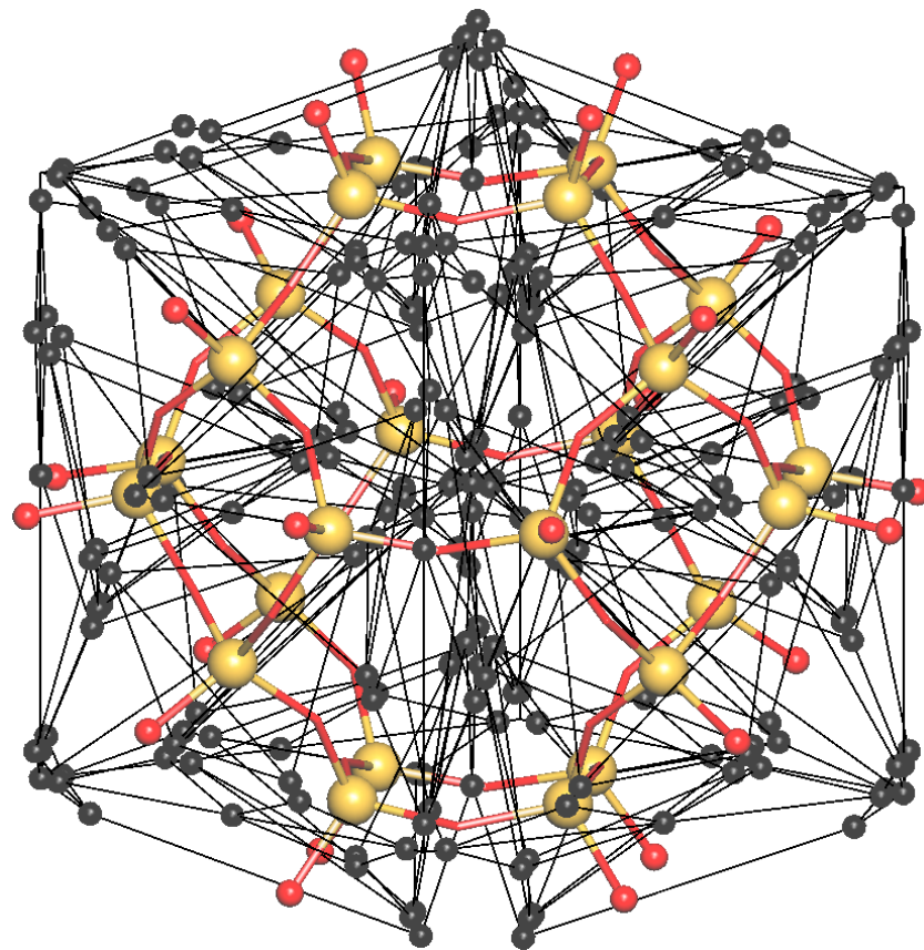
Сетка Вороного для содалитного каркаса
