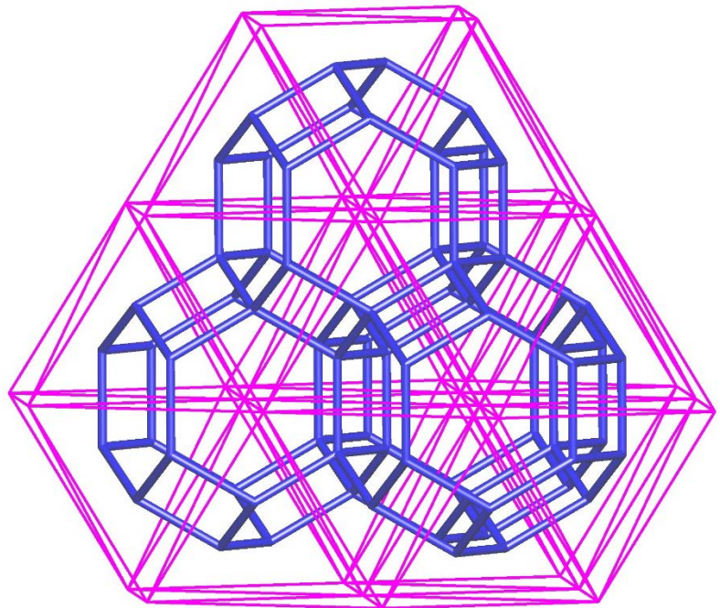
Дуальная сетка тайлинга 24/14:[4^6.6^8] - bcsu-x
