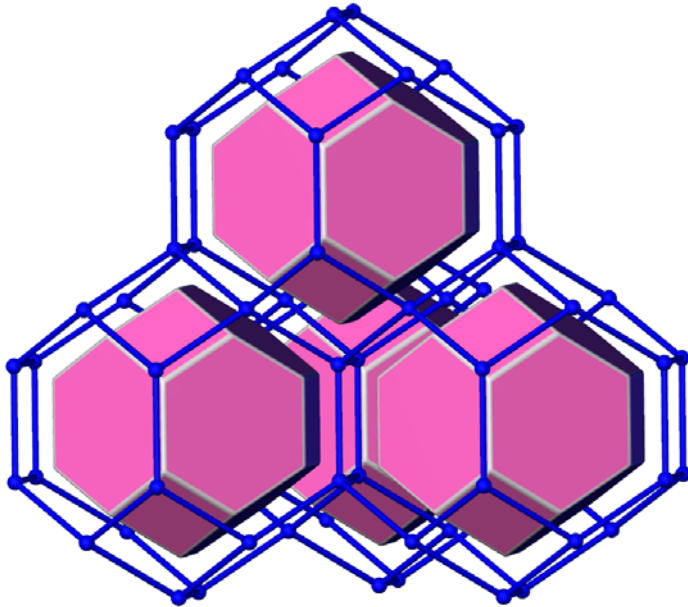
Топологический мотив каркаса содалита sod и его тайлинг 24/14:[4^6.6^8]
