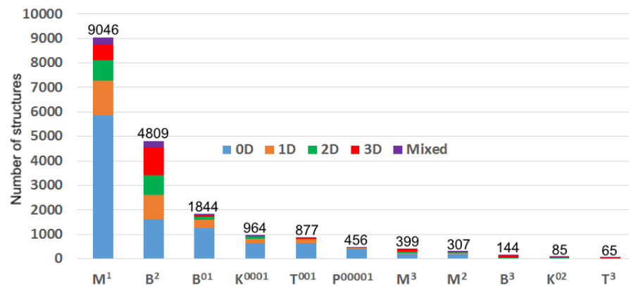
Координация лигандов
