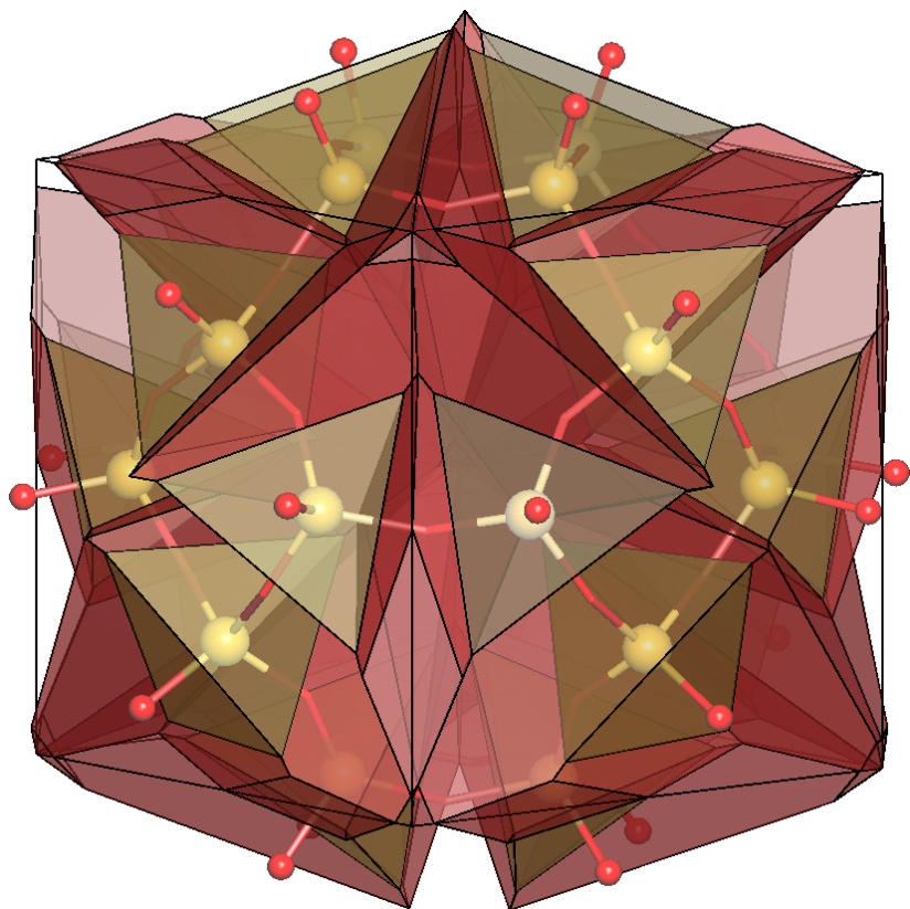
Разбиение Вороного
