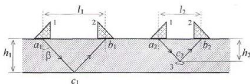
Рис. 3. Определение глубины дефекта с помощью акустических волн: 1 – источник, 2 – приемник, 3 – возможный дефект
