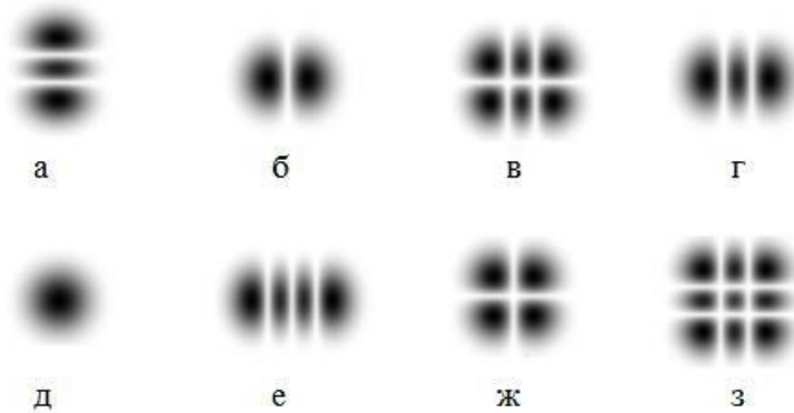
Рисунок 1 – Поперечные моды оптического резонатора
