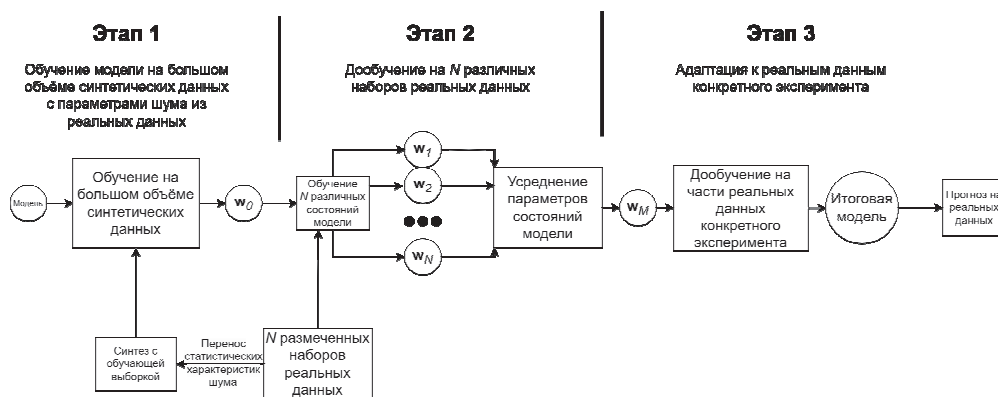
Рис. 2. Схема алгоритма метаобучения моделей обнаружения аномалий с использованием синтетических данных. w_0 – вектор параметров начального состояния нейросетевой модели, N – количество реальных сигналов первого измерения и количество получаемых на втором этапе состояний модели, w_1 \dots w_N – набор параметров модели после дообучения из начального состояния, w_M – результирующий набор параметров модели
