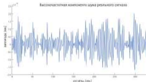
Рис. 4. Высокочастотный шум, извлечённый из реального сигнала с помощью дискретного вейвлет-преобразования
